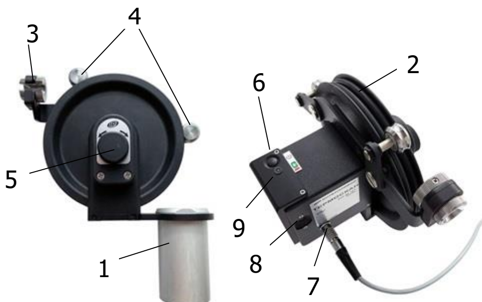
Рисунок 3 – Энкодер
