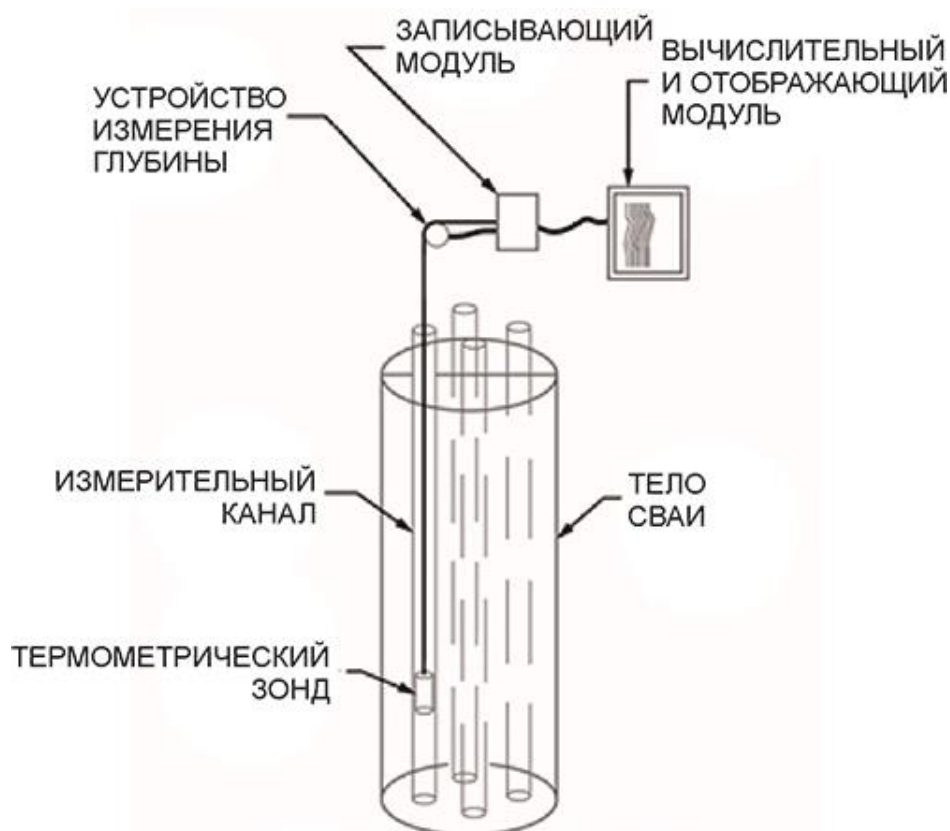
Рисунок 1 – Схема измерения
