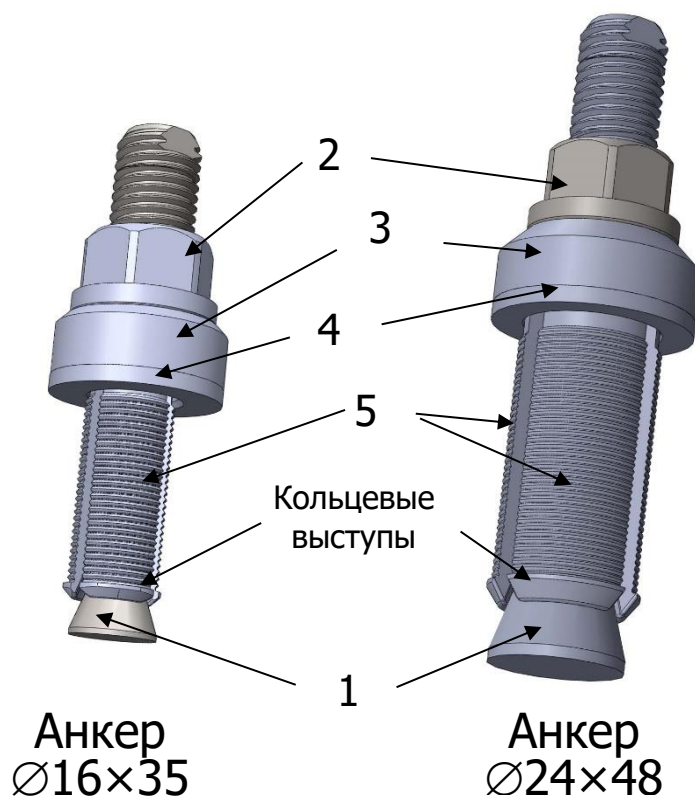
Рисунок 3 – Анкерные устройства (анкера) в сборе
