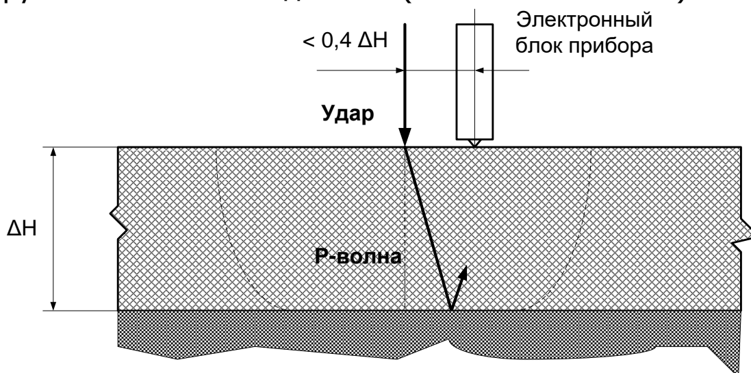
Рисунок 6 – Ориентация ударного элемента и электронного блока прибора при измерениях
