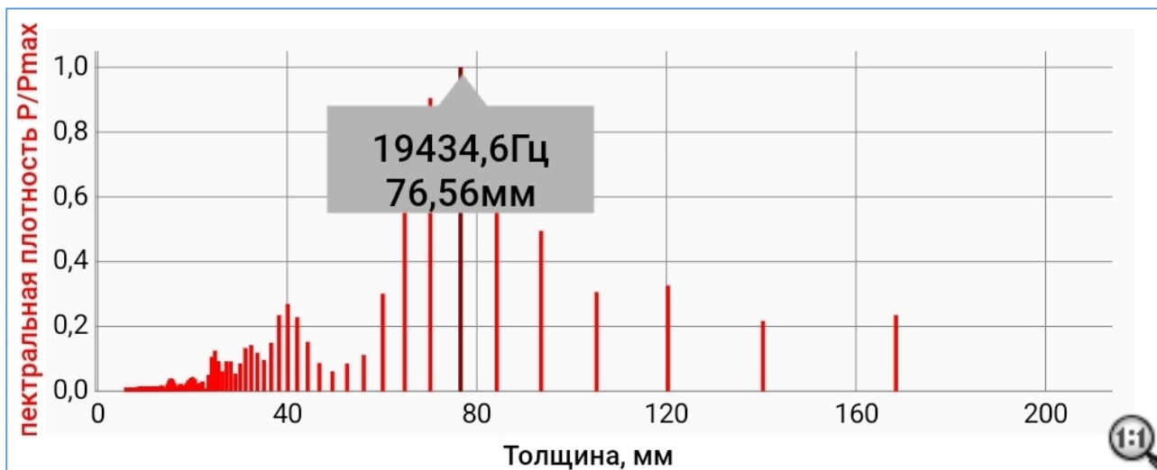
Рисунок 22 – Итоговая спектральная характеристика P(H)
