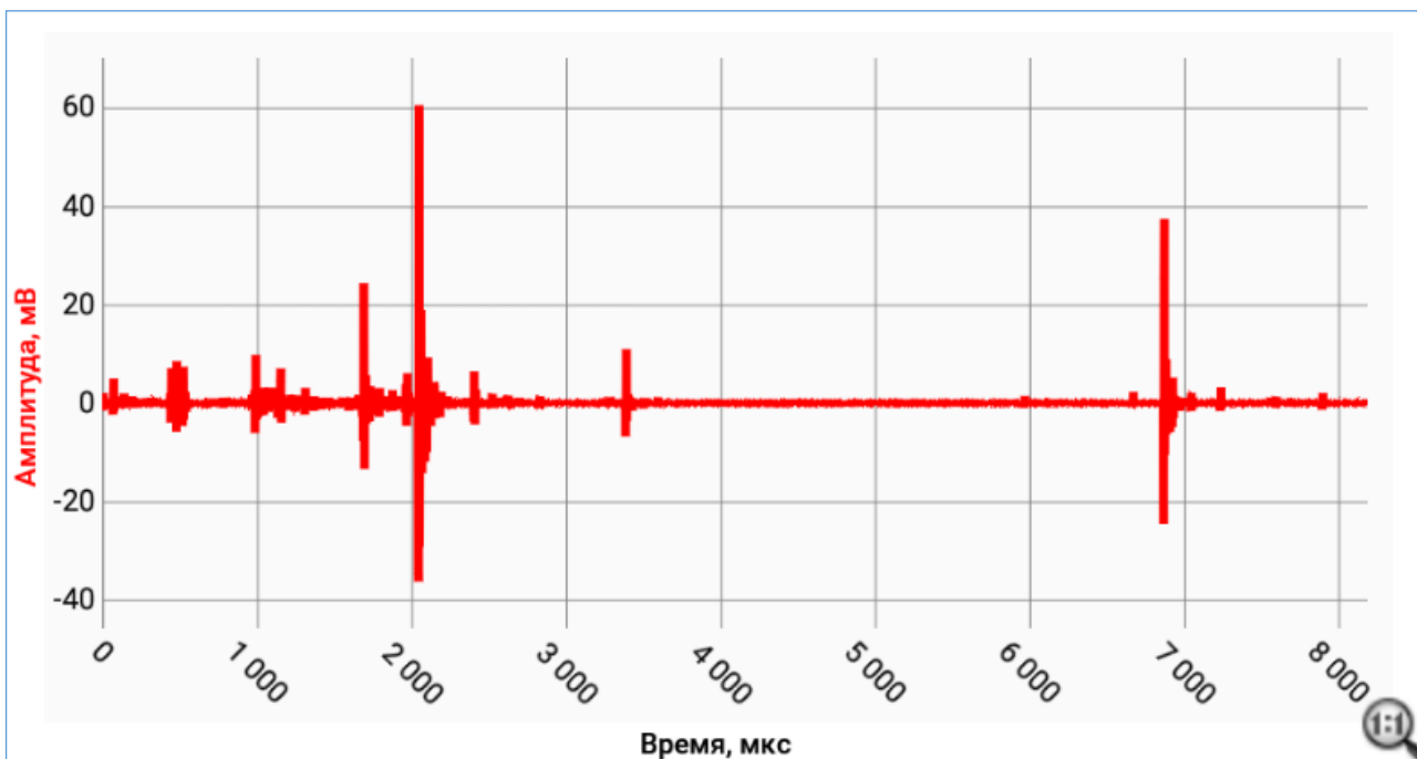
Рисунок 7 – Пример некорректного сигнала с удаленной постоянной составляющей
