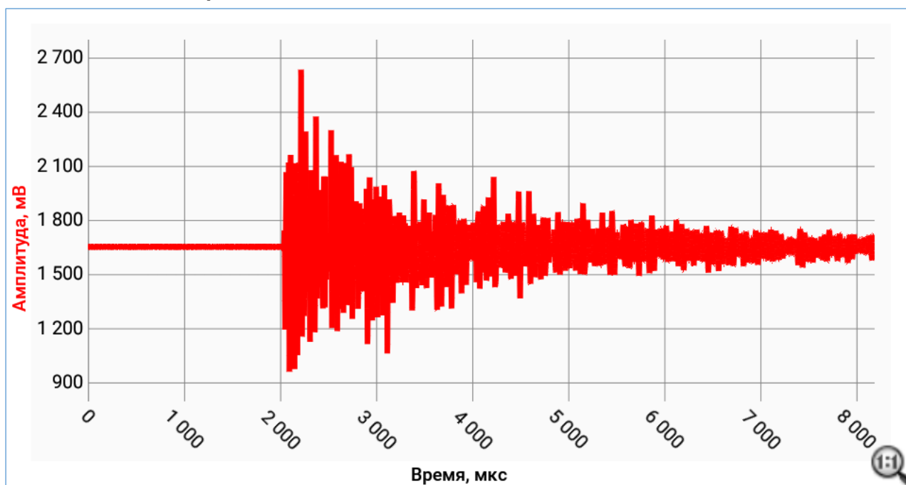
Рисунок 8 – Пример корректного сигнала
