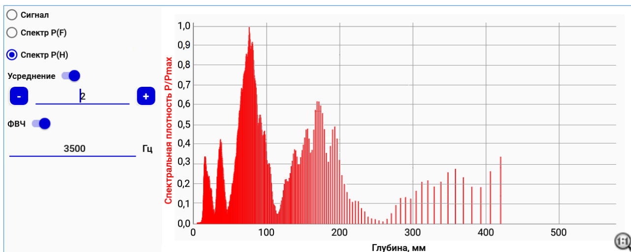
Рисунок 17 – Спектральная характеристика сигнала с определением толщины объекта по максимальному соотношению P/P_{max} и применением ФВЧ
