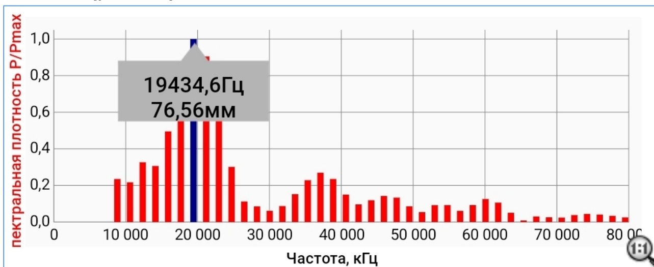
Рисунок 21 – Спектральная характеристика захваченного участка временной диаграммы после применения ФВЧ 10 кГц
