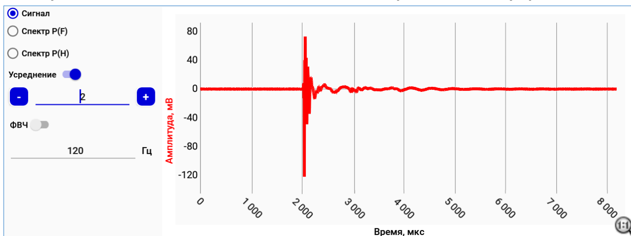
Рисунок 14 – Сигнал с применением усреднения N=2
