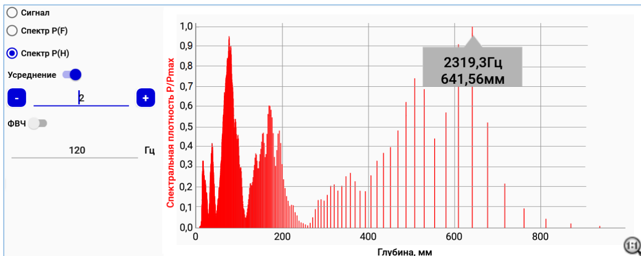
Рисунок 15 – Спектральная характеристика сигнала с определением толщины объекта по максимальному соотношению P/P_{max} (вид – первый максимум с/плотности)
