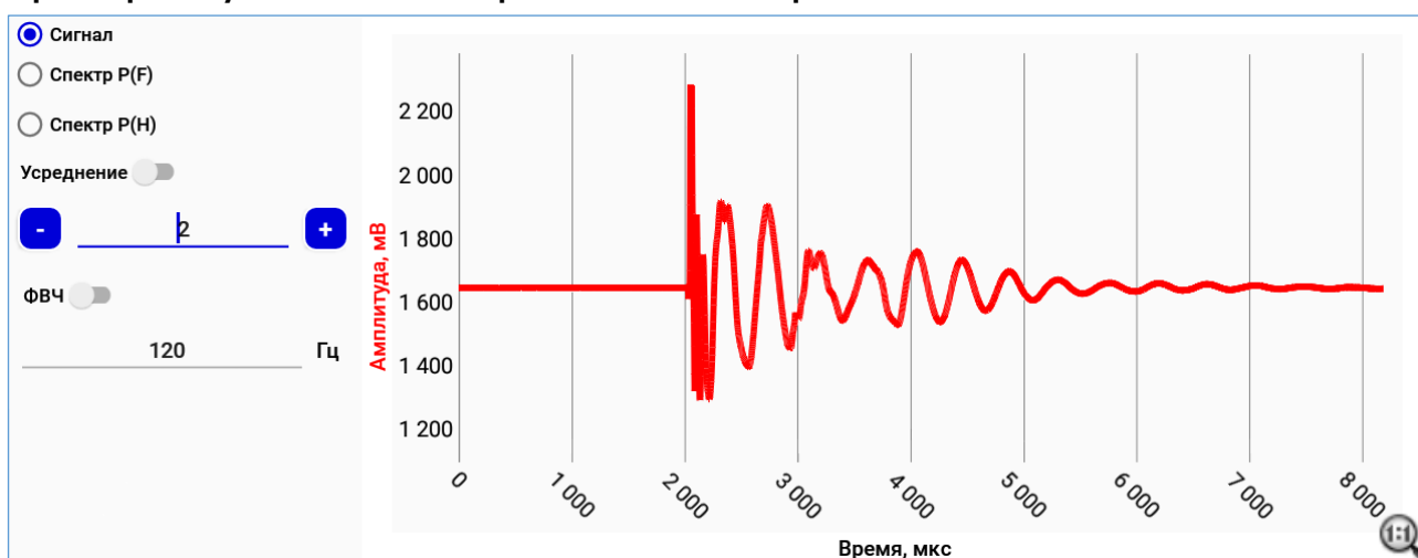
Рисунок 13 – Изначальный сигнал до применения усреднения
