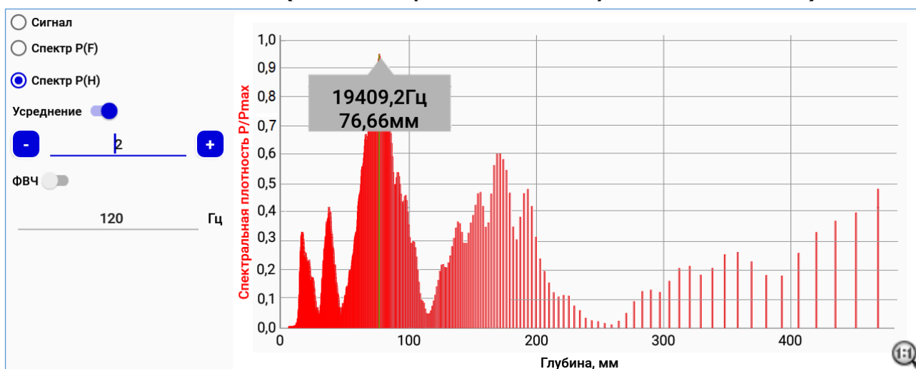
Рисунок 16 – Спектральная характеристика сигнала с определением толщины объекта по максимальному соотношению P/P_{max} (вид – второй максимум с/плотности)
