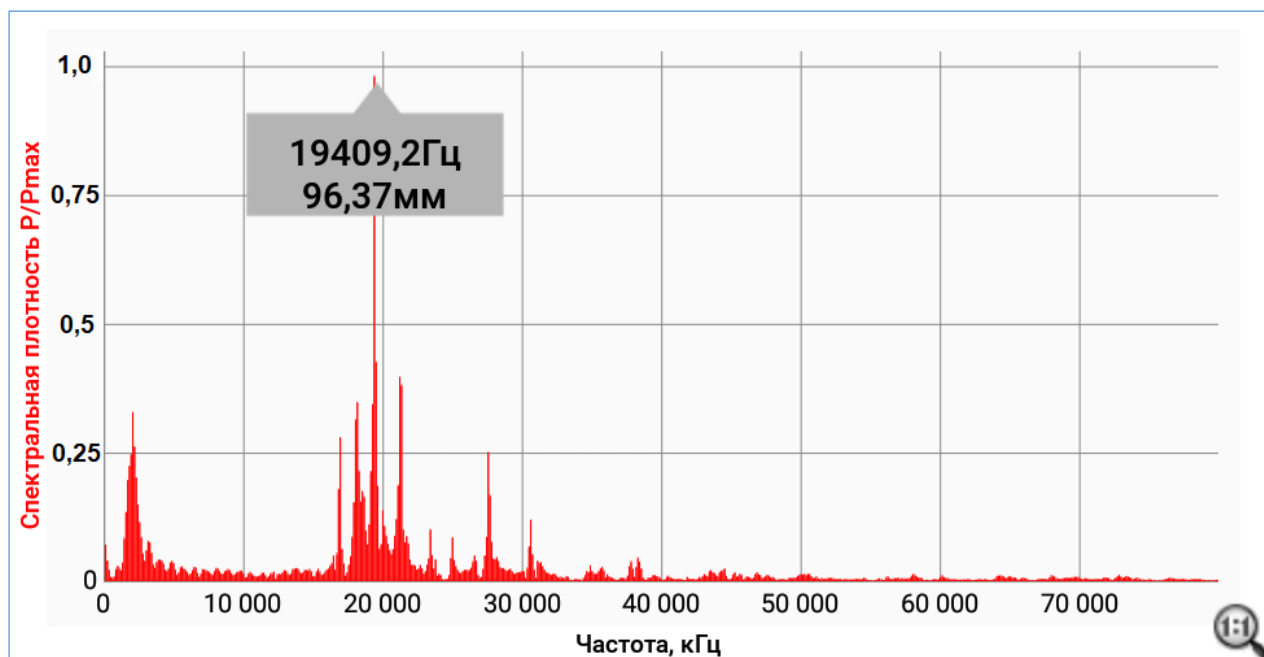
Рисунок 10 – Спектральная частотная характеристика сигнала
