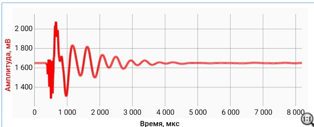
Рисунок 18 – Исходная амплитудная характеристика измеренного сигнала
