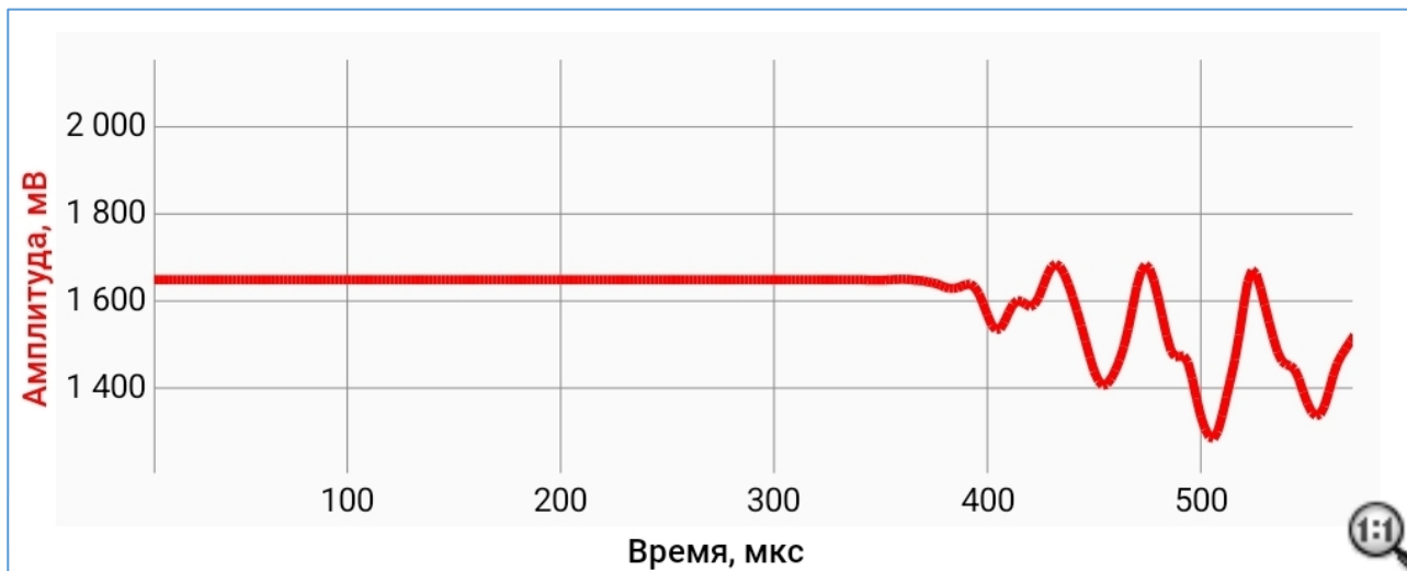
Рисунок 19 – Захваченный участок временной диаграммы
