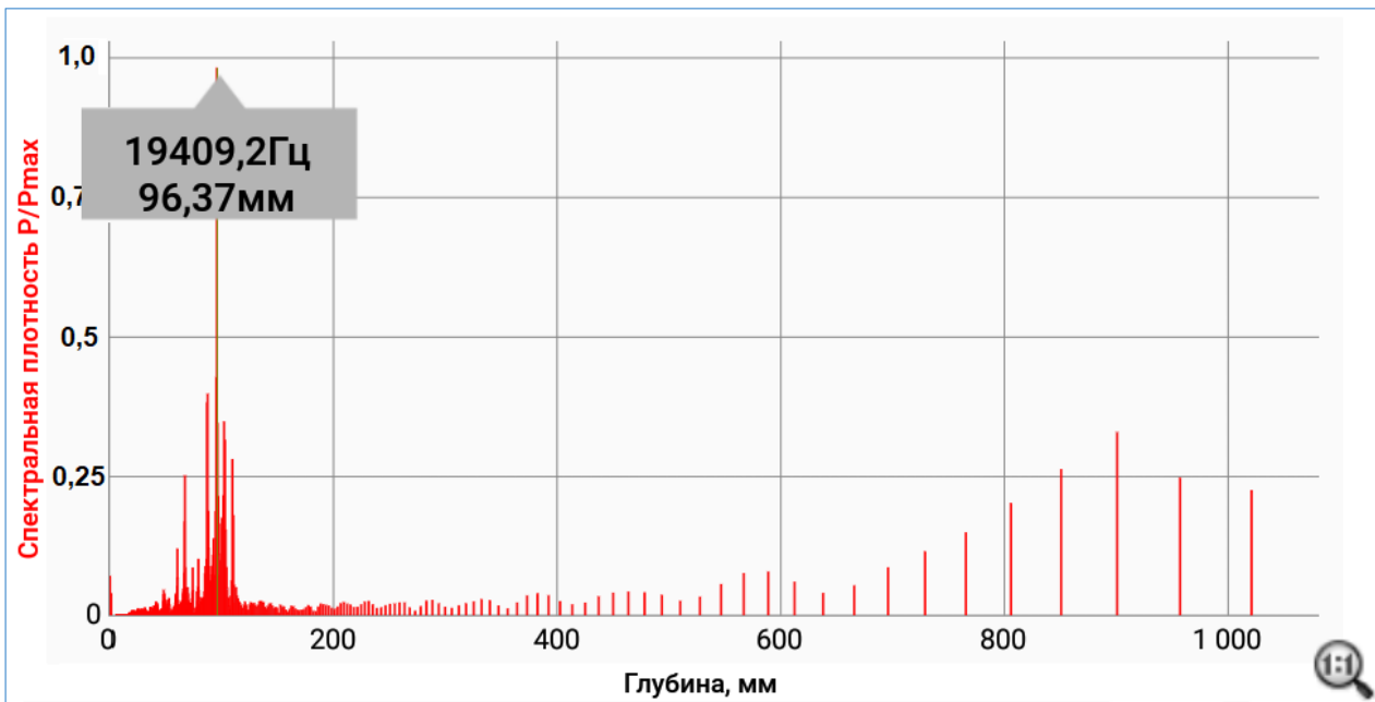
Рисунок 11 – Спектральная частотная характеристика сигнала с определением толщины объекта по максимальному соотношению P/P_{max}
