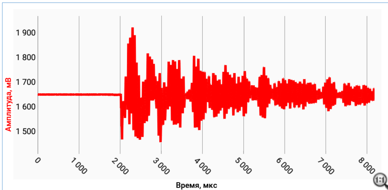
Рисунок 9 – Временная характеристика сигнала, Объект – Куб 100 мм
