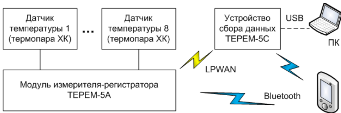
Рисунок 1 - Структурная схема внешних связей устройств системы контроля
