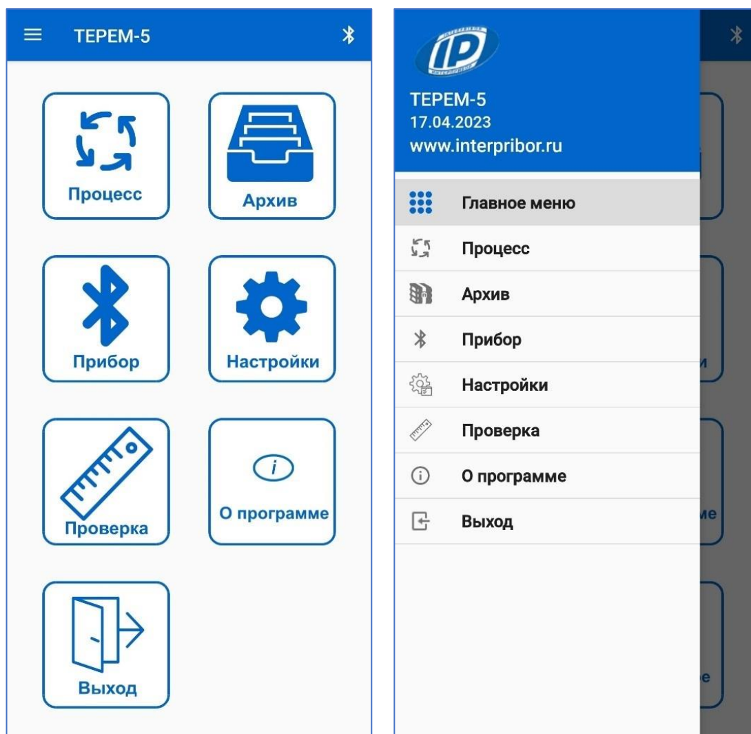
Рисунок 5 – Главное меню
