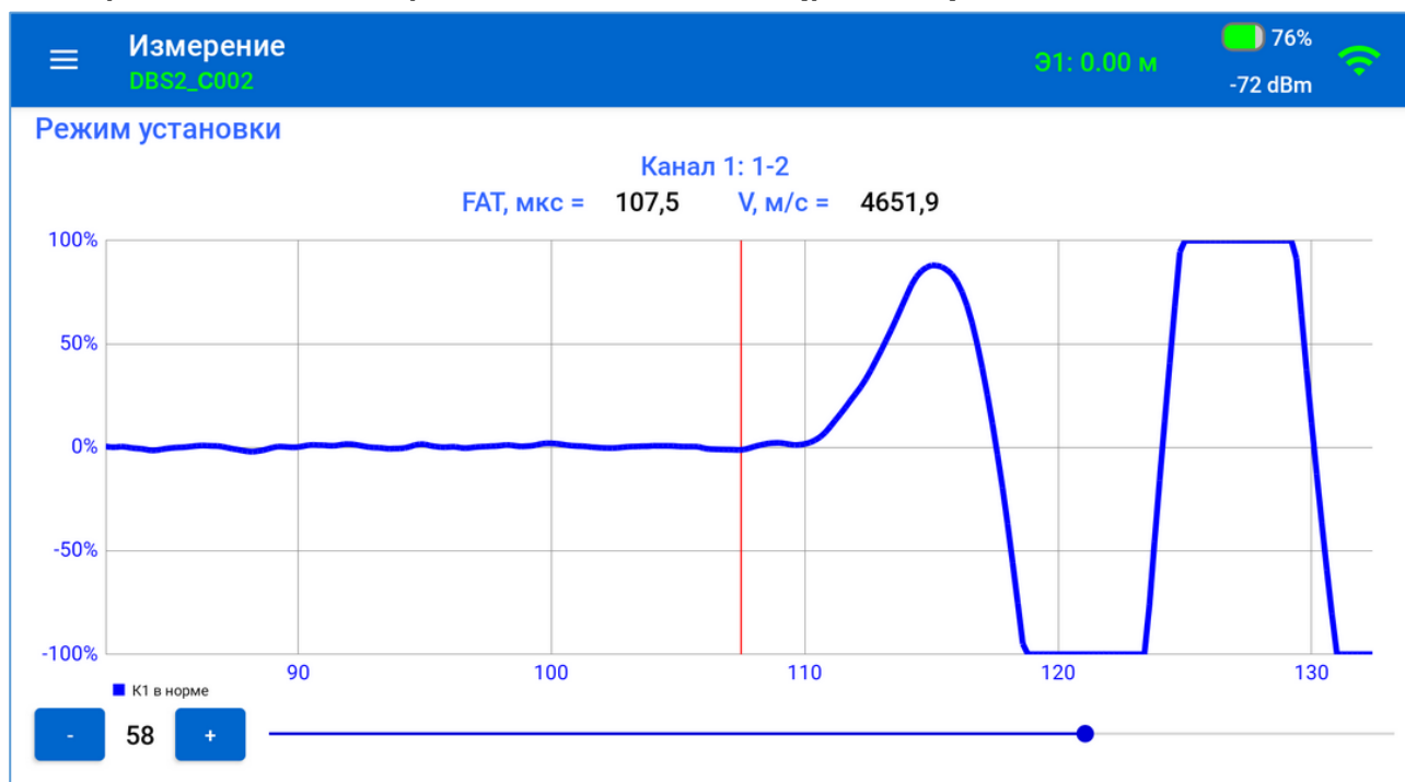
Рисунок 45 – Экран «Измерение», режим настройки усиления сигналов от УЗ зондов
