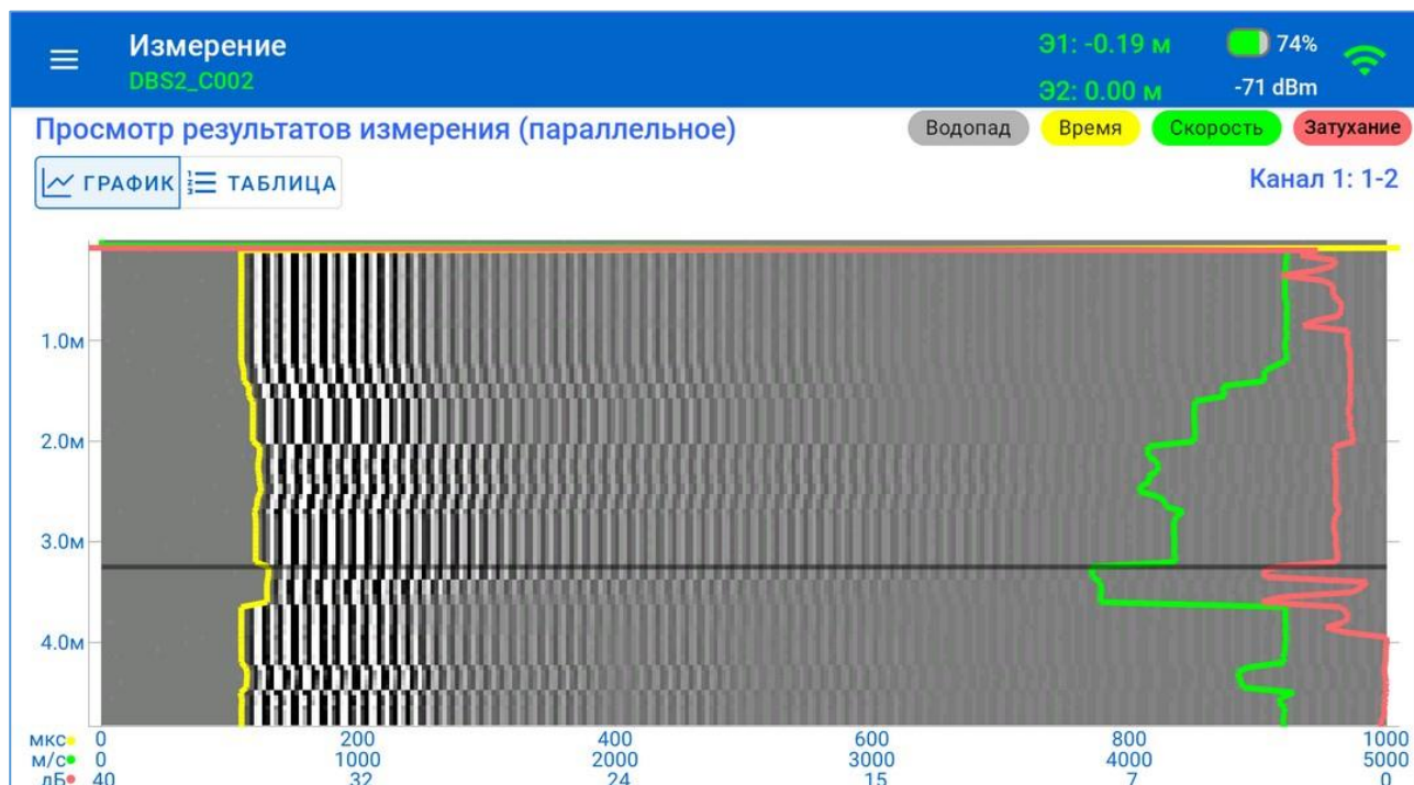
Рисунок 29 – Экран вывода архивных результатов измерений
