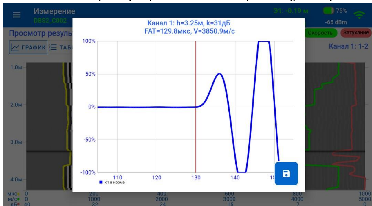
Рисунок 30 – Экран вызова числовых значений и графика зарегистрированного УЗ сигнала в произвольном месте диаграммы
