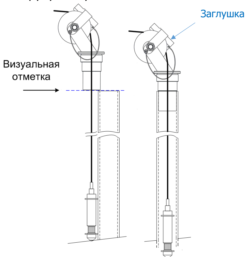
Рисунок 43 – Размещение зонда в трубе доступа на уровне поверхности бетона
