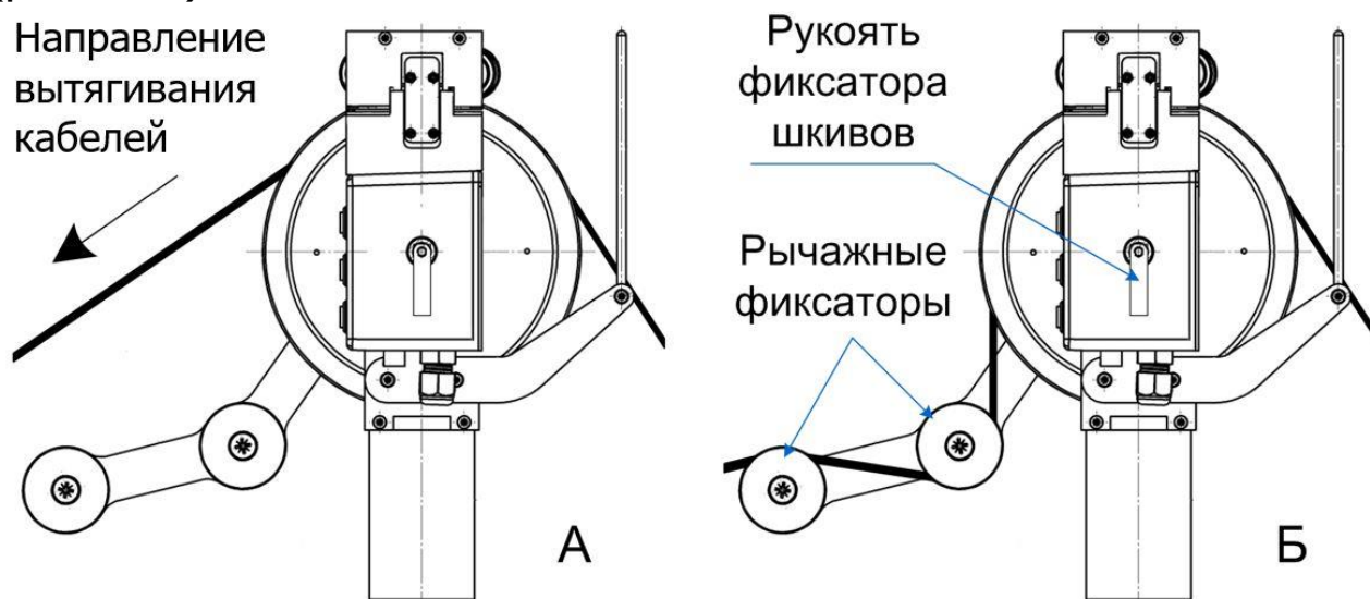
Рисунок 44 – Заправка кабеля за фиксаторы кабелей БЭ
