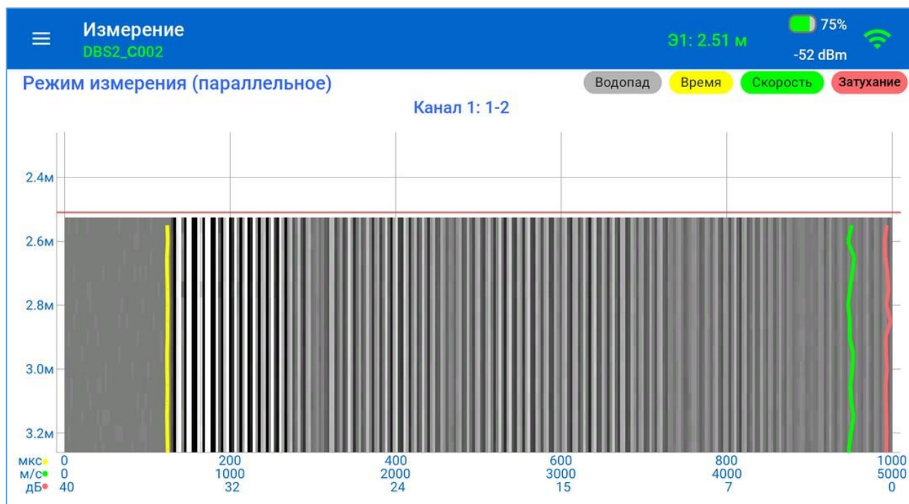
Рисунок 27 – Экран «Измерение», режим измерений
