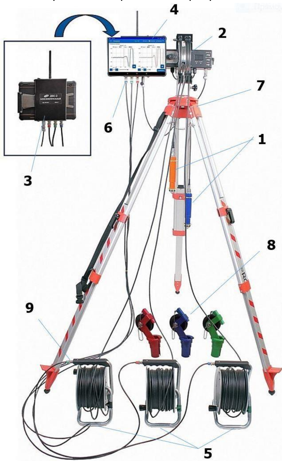
Рисунок 3 – Установка ДБС-2 в сборе
