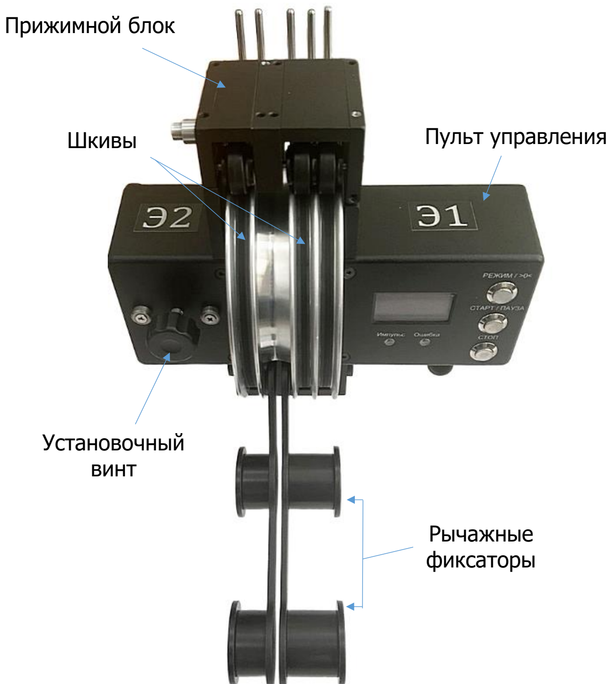
Рисунок 6 – Блок энкодеров установки ДБС-2
