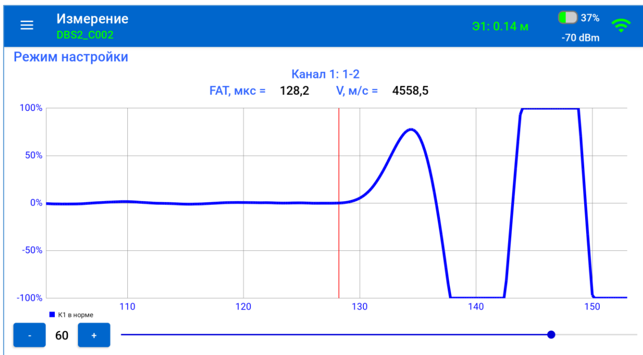
Рисунок 25 – Экран «Измерение», режим настройки усиления
