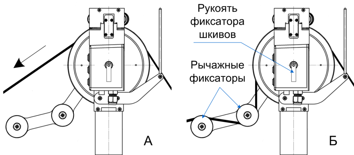
Рисунок 43 – Заправка кабеля за фиксаторы кабелей БЭ
