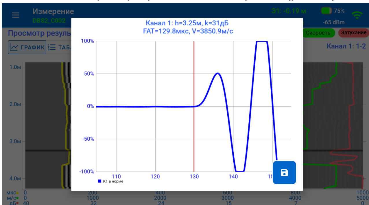
Рисунок 29 – Экран вызова числовых значений и графика зарегистрированного УЗ сигнала в произвольном месте диаграммы
