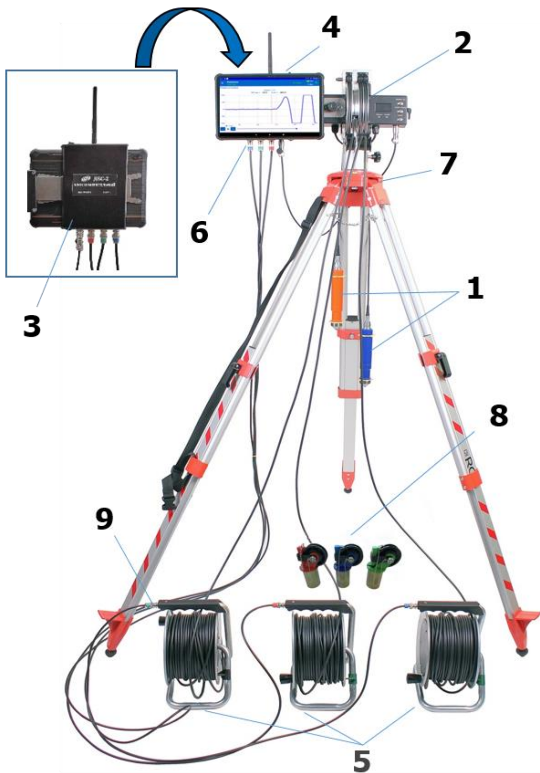
Рисунок 3 – Установка ДБС-2 в сборе
