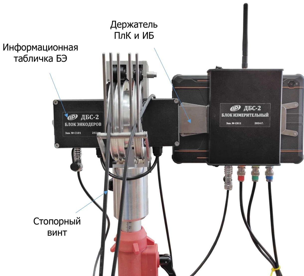
Рисунок 40 – Установка БЭ, ИБ и ПЛК на штатив (вид на БЭ сзади)
