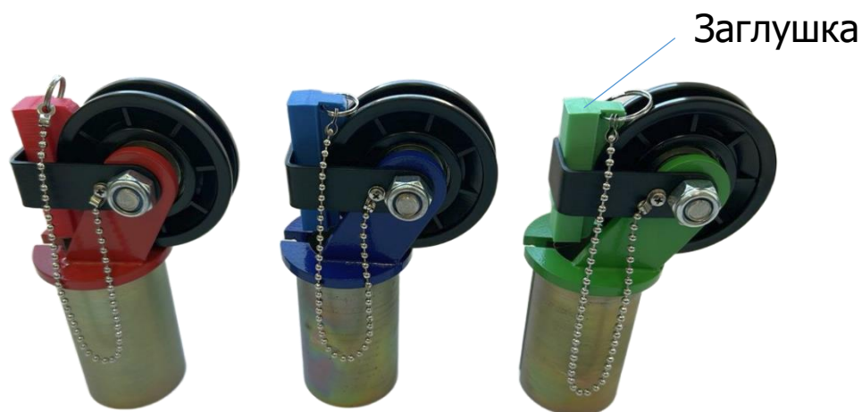
Рисунок 5 – Установочные втулки для протягивания кабеля зонда
