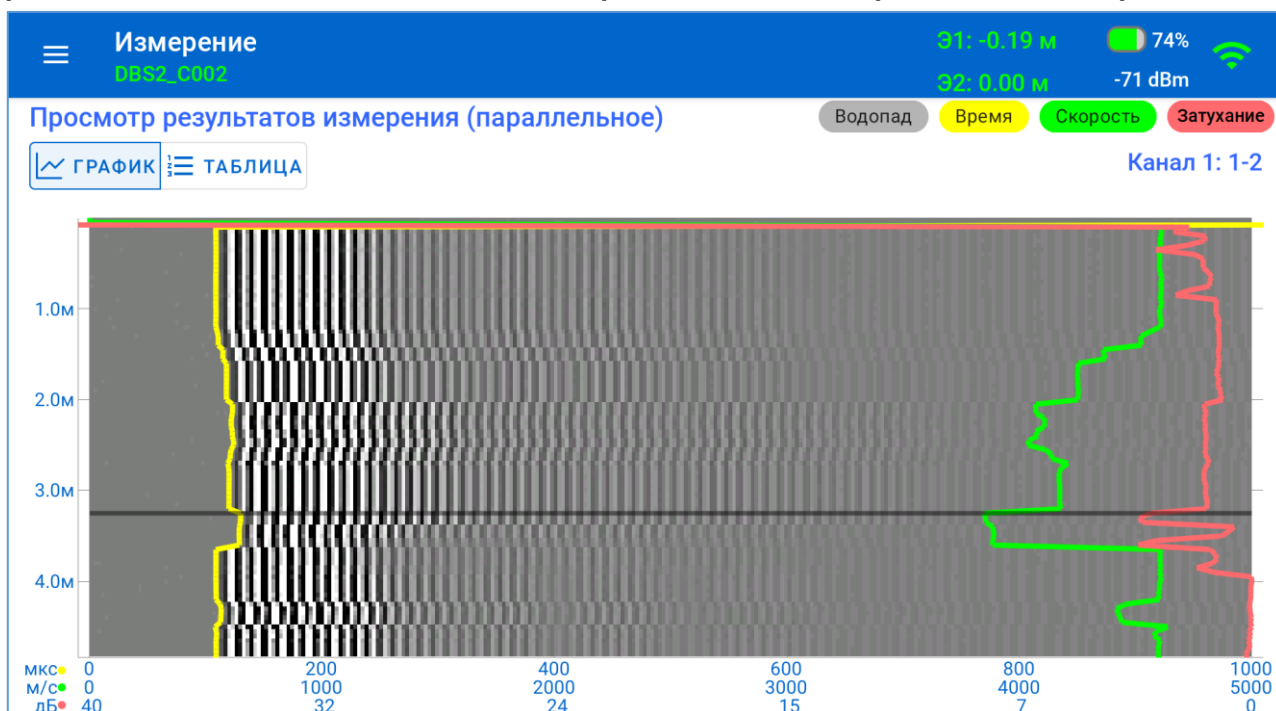
Рисунок 28 – Экран вывода архивных результатов измерений
