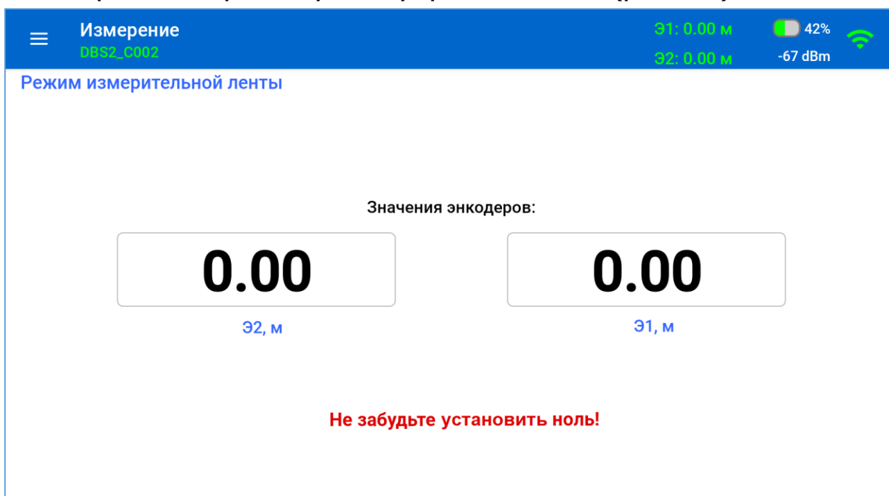
Рисунок 24 – Экран «Измерение, режим измерительной ленты
